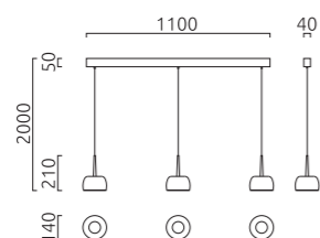
19 W, 2800 K, B 2140 / N 1320 lm, CRI > 90 36/2002.04
