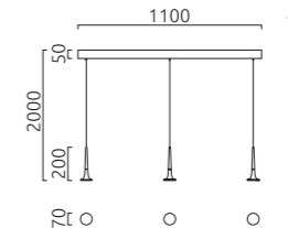
19 W, 2800 K, B 2140 / N 1320 lm, CRI > 90 36/2002.04
